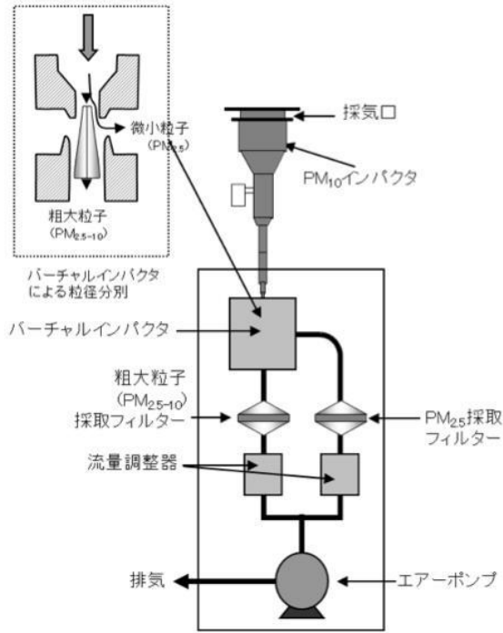
図3 FRMサンプラー装置の概略例
