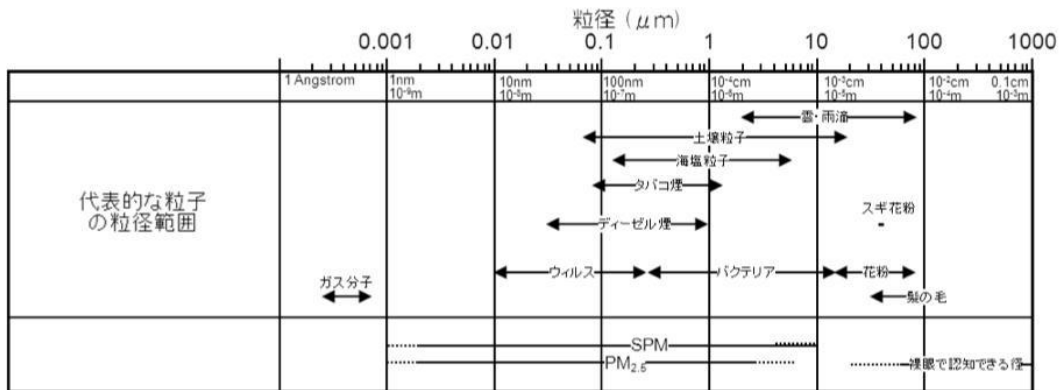
図1 代表的な粒子状物質の粒径 (出典：William C. Hinds, 1999, Aerosol Technology, A Wiley-Interscience Publication 原図を巻末に記す。土壌粒子、海塩粒子の粒径範囲は、外山敏夫1985から追記。)
